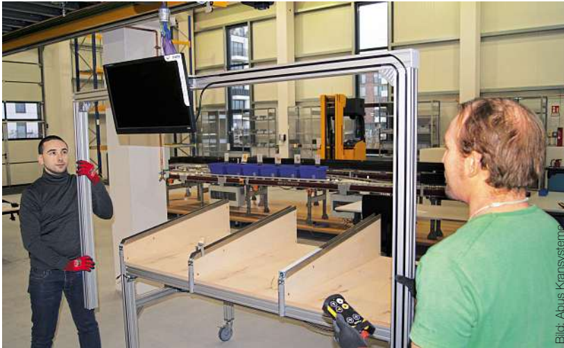
Die Hängebahnanlage unterhalb der Stahlbühne im Versuchsfeld bietet Unterstützung bei leichten Handling-Aufgaben, hier zum Beispiel bei der Montage eines Kommissioniertisches.
