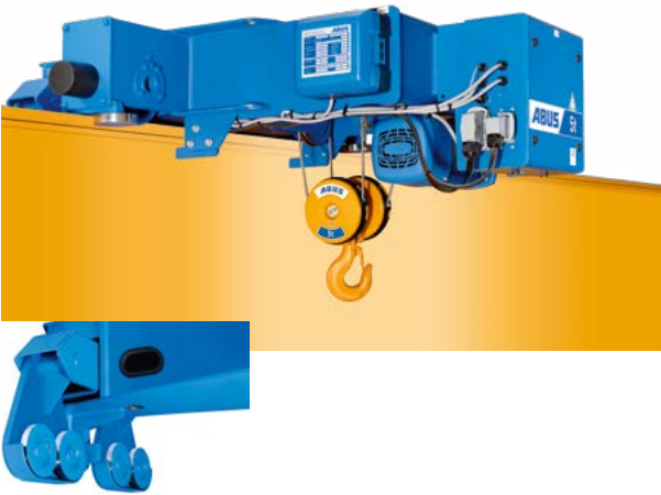
Stützrollen mit Drehgelenk
